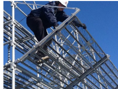
④ 隣接したスパンに同様の手順で取り付け、踏板を手前から設置する
